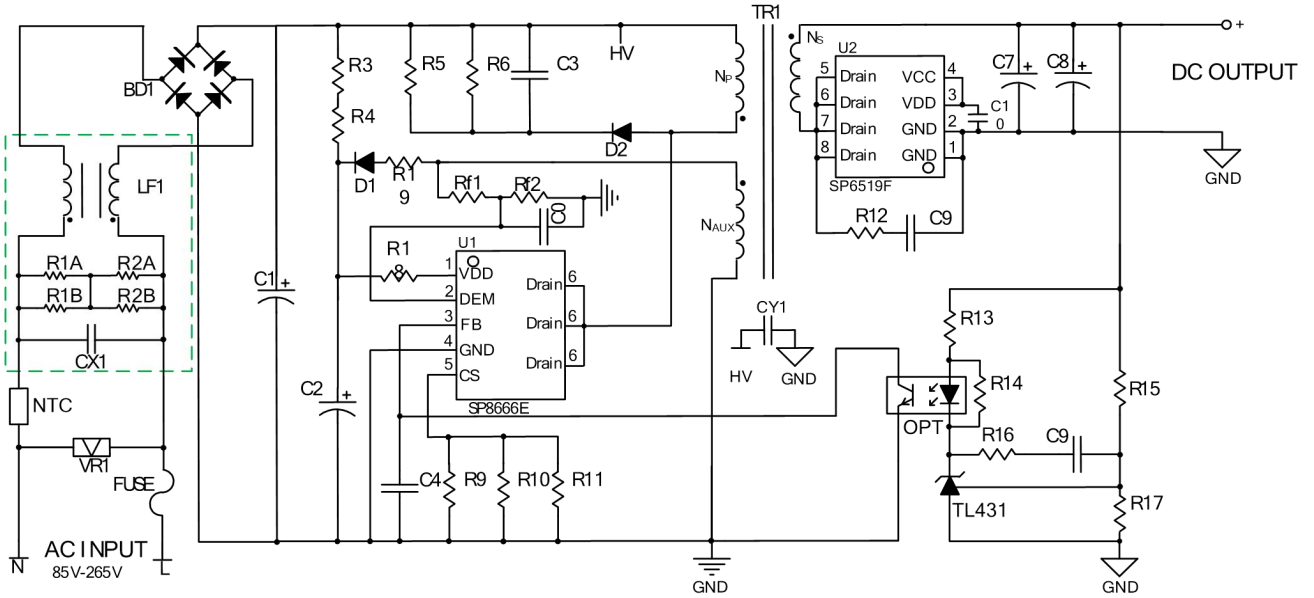
图 1 典型应用图
